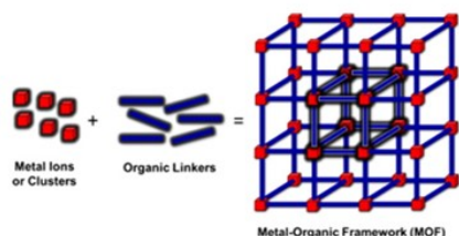
Figura 1: Formación de MOFs por iones metálicos o cúmulos y enlazadores orgánicos.
